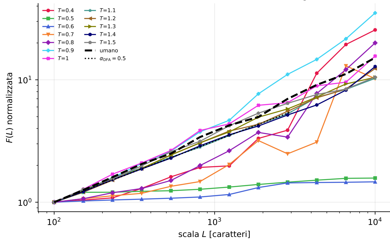
DFA sui caratteri — Qwen3.5-4B-Base (cfr. [L] Fig. 4A)
